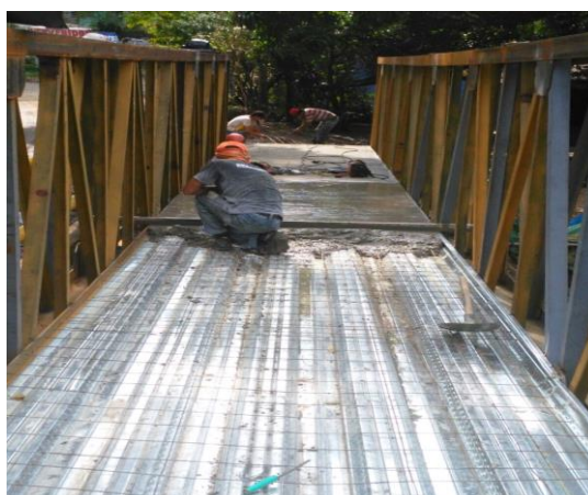
Imagen 12. Placa de metaldeck.
