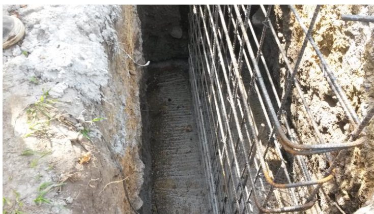
Imagen 8. Fundida con concreto clase D 4000 PSI para la zapata #1.
