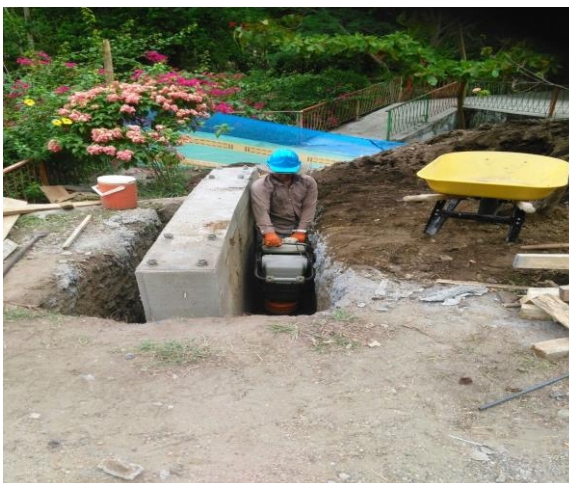
Imagen 7. Compactación del material.
