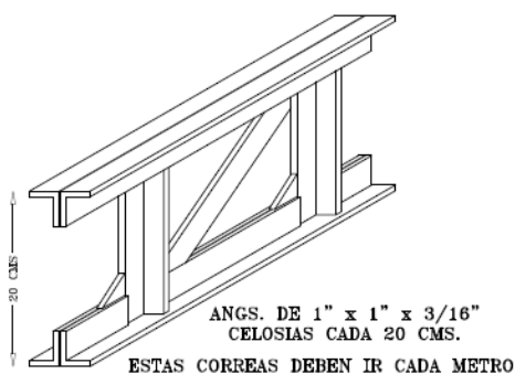
DETALLE CORREA METALICA (PARA APOYO DE PACA) ESCALA: 1:10
