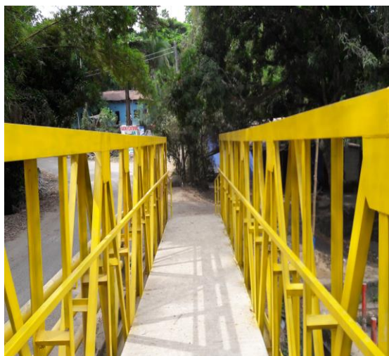
Imagen 20. Angulo longitudinal de 5" x 5" x 3/8".
