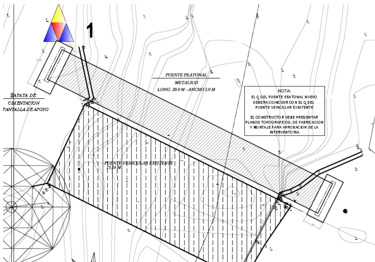
Imagen 1. Plano en formato PDF, entregado por la gobernación del Tolima
